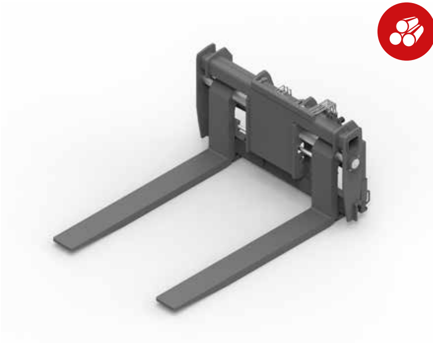
FCEP30T 2,4 R
